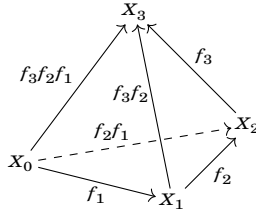
FIG. 4.1. : Représentation graphique d'un élément de N_3 \mathbf{C}
