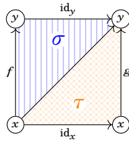
FIG. 4.4. : Représentation d'un élément de \text{Map}_{\mathcal{C}}(x, y)_1
