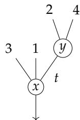
FIG. 4.4 : Un élément de WD_n , où x \in D_n(3) , y \in D_n(2) et t \in [0, 1] .
