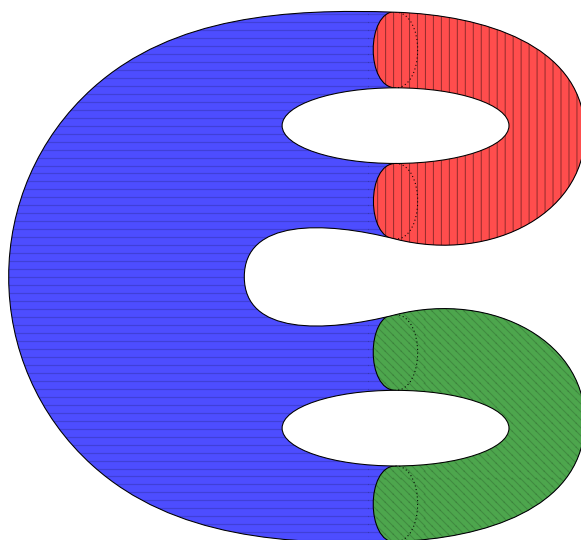
FIG. 3.1 : La surface \Sigma_2 obtenue en recollant une sphère à quatre trous (bleue) avec deux cylindres (rouge et vert).
