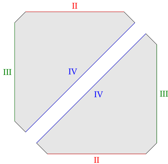
FIG. 3.8 : L'espace \mathfrak{mFM}_{[0,1]}(2) et ses strates de codimension 1. Les petits segments (en noir) font tous partie de la strate V.
