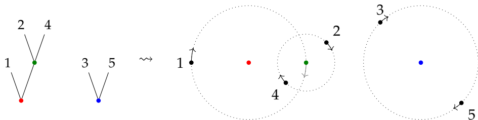
FIG. 1.7 : Systèmes solaires : un arbre à 5 feuilles et 3 sommets internes induit une classe d'homologie dans H_{3(n-1)}(\text{Conf}_{\mathbb{R}^n}(5)) ; ici, n = 2 .
