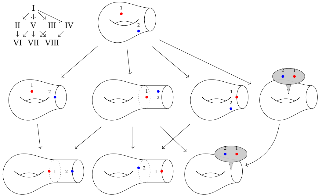
FIG. 3.6 : Strates de mFM_M(2) .
